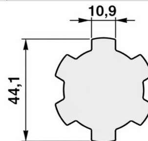
1"3/4 Z=6
