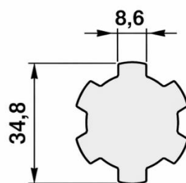
1"3/8 Z=6
