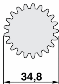
1"3/8 Z=21
